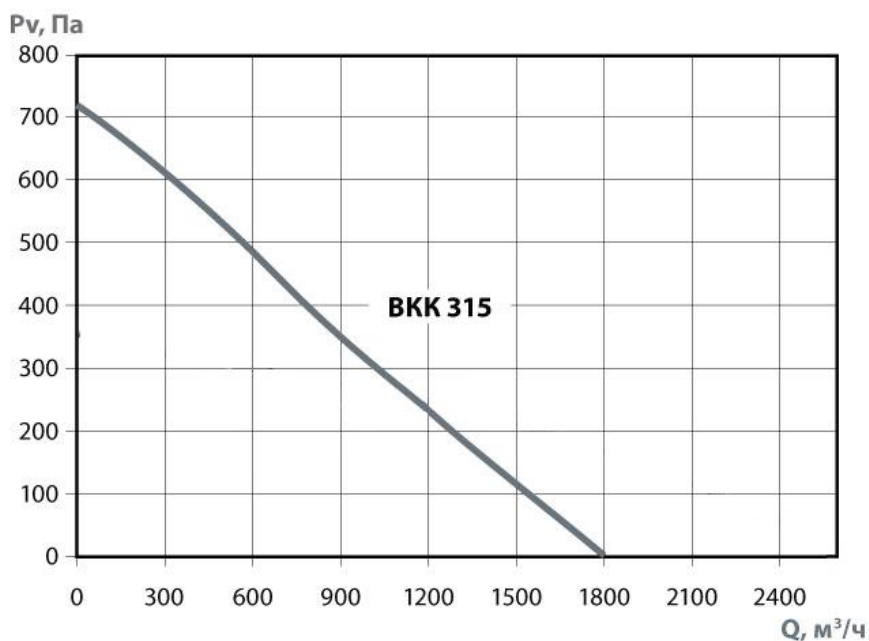
Аэродинамическая характеристика вентилятора ВКК 315
