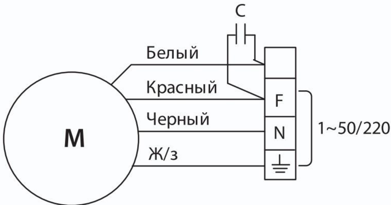
РИС. 2. Схема подключения вентиляторов ВКК
