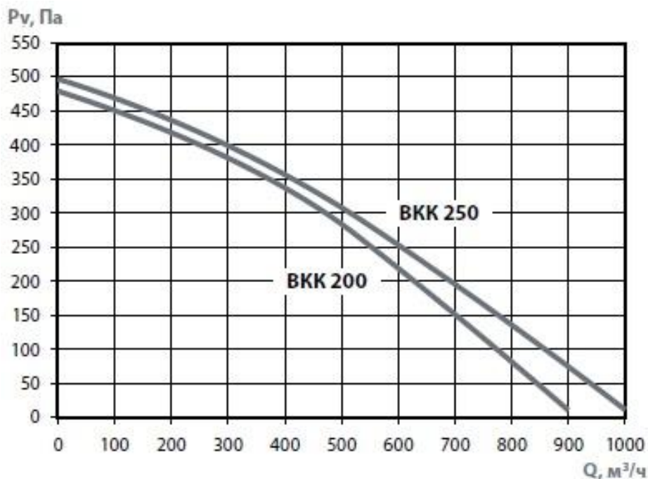
Аэродинамическая характеристика вентиляторов ВКК 200, 250
