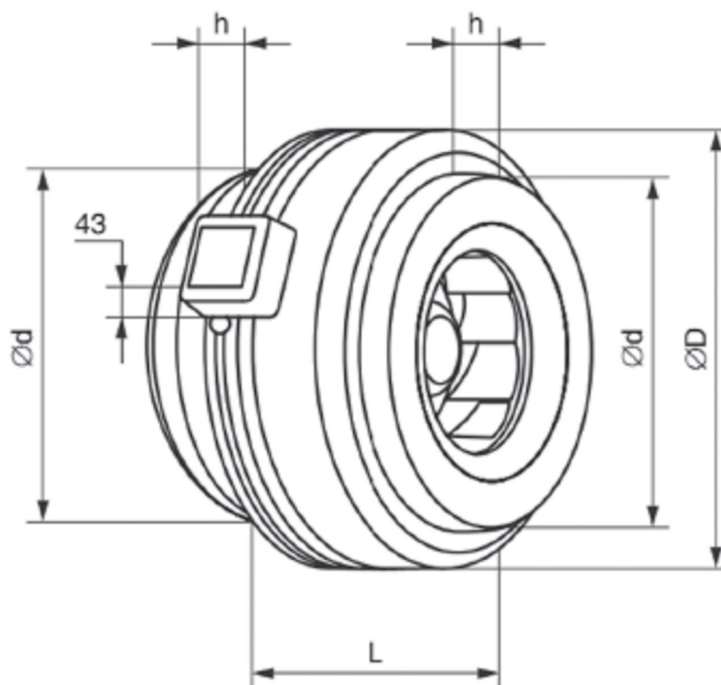
РИС. 1. Габаритные и присоединительные размеры вентиляторов ВКК
